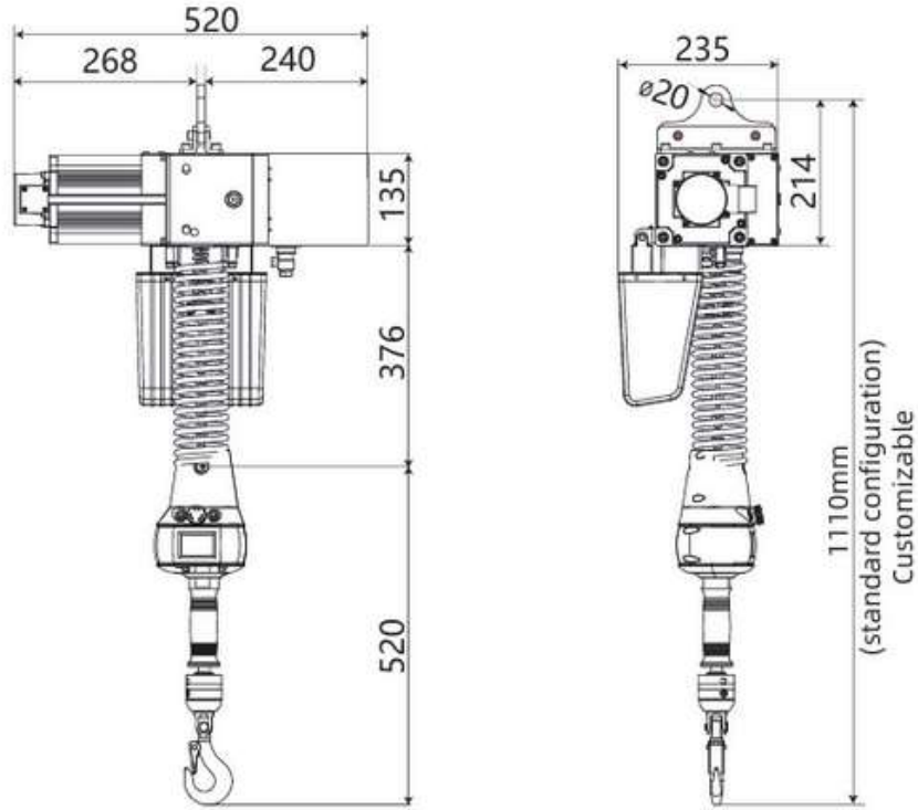
ST11-100/ST11-200 Serisi Ürün Boyutu
