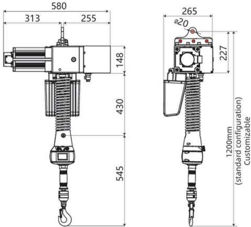
ST11-300/ST11-500 Serisi Ürün Boyutu
